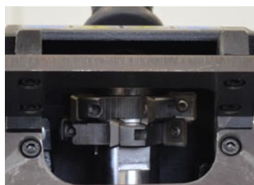
2 forgó marófej, egyenként öt négyoldalú forgatható betéttel
