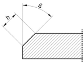
1. rajz Vágási méretek: max. vágási szélesség a szögtől függően
