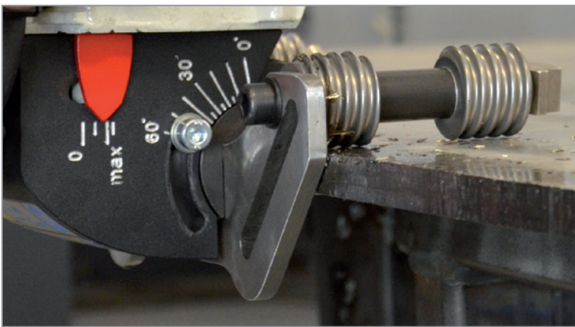
Fokozatmentes leélezési szögbeállítás 0°-tól 60°-ig
